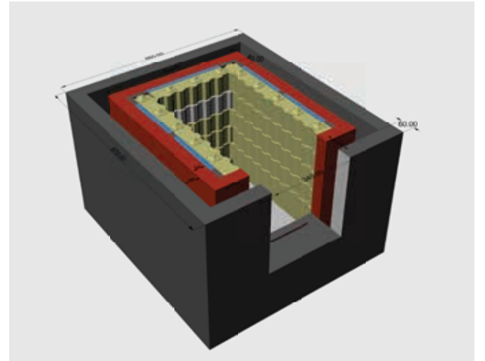
Ahju koldehisu element – õhuvahe, kolde välissein ja ahju väliskest.
